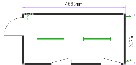
16-и футовый офисный блок-контейнер
